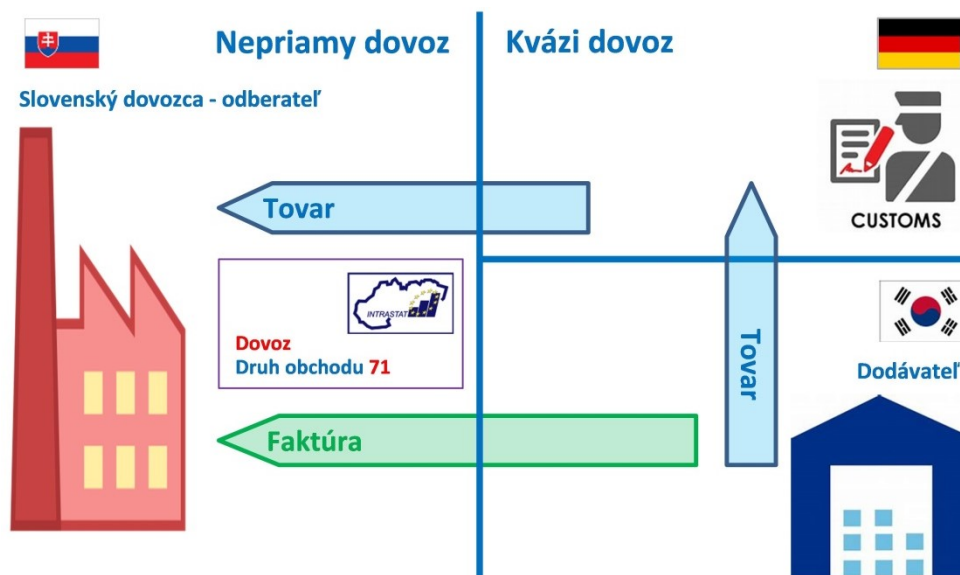
Obrázok 26: Nepriamy dovoz
