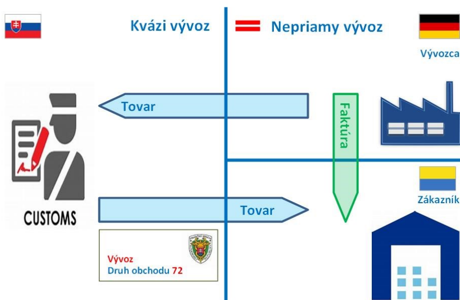
Obrázok 3: Kvázivývoz
